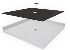
TileOver
